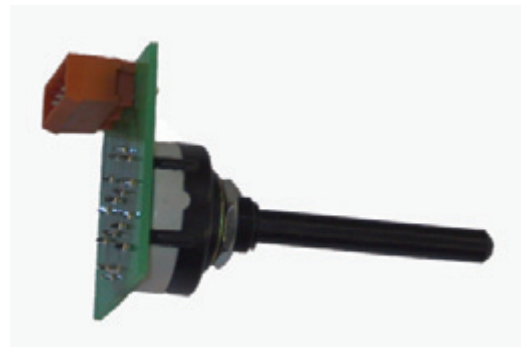
Circuit imprimé commutateur changement de vitesse hydraulique Commutator of change of hydraulic speed printed circuit Ref 007 084 000
