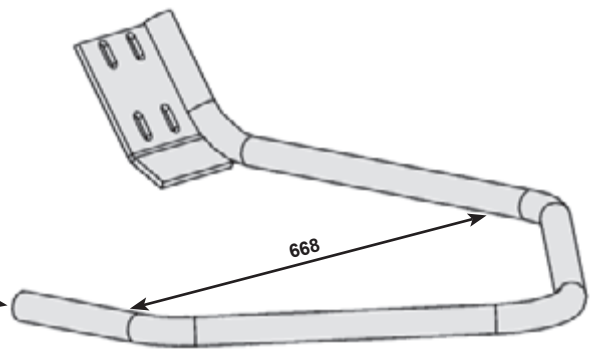
Diviseur droit large Large right divider 241 136 000
