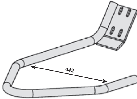
Diviseur gauche Left divider 241 135 000
