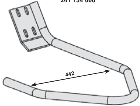
Diviseur droit Right divider 241 134 000
