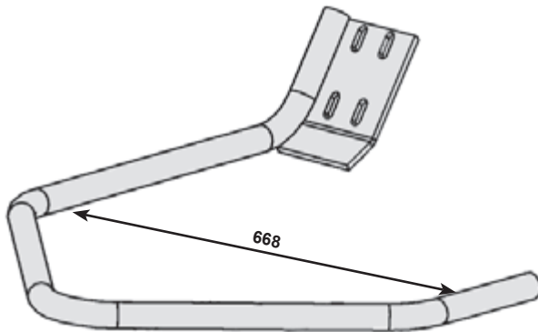
Diviseur gauche large Large left divider 241 137 000
